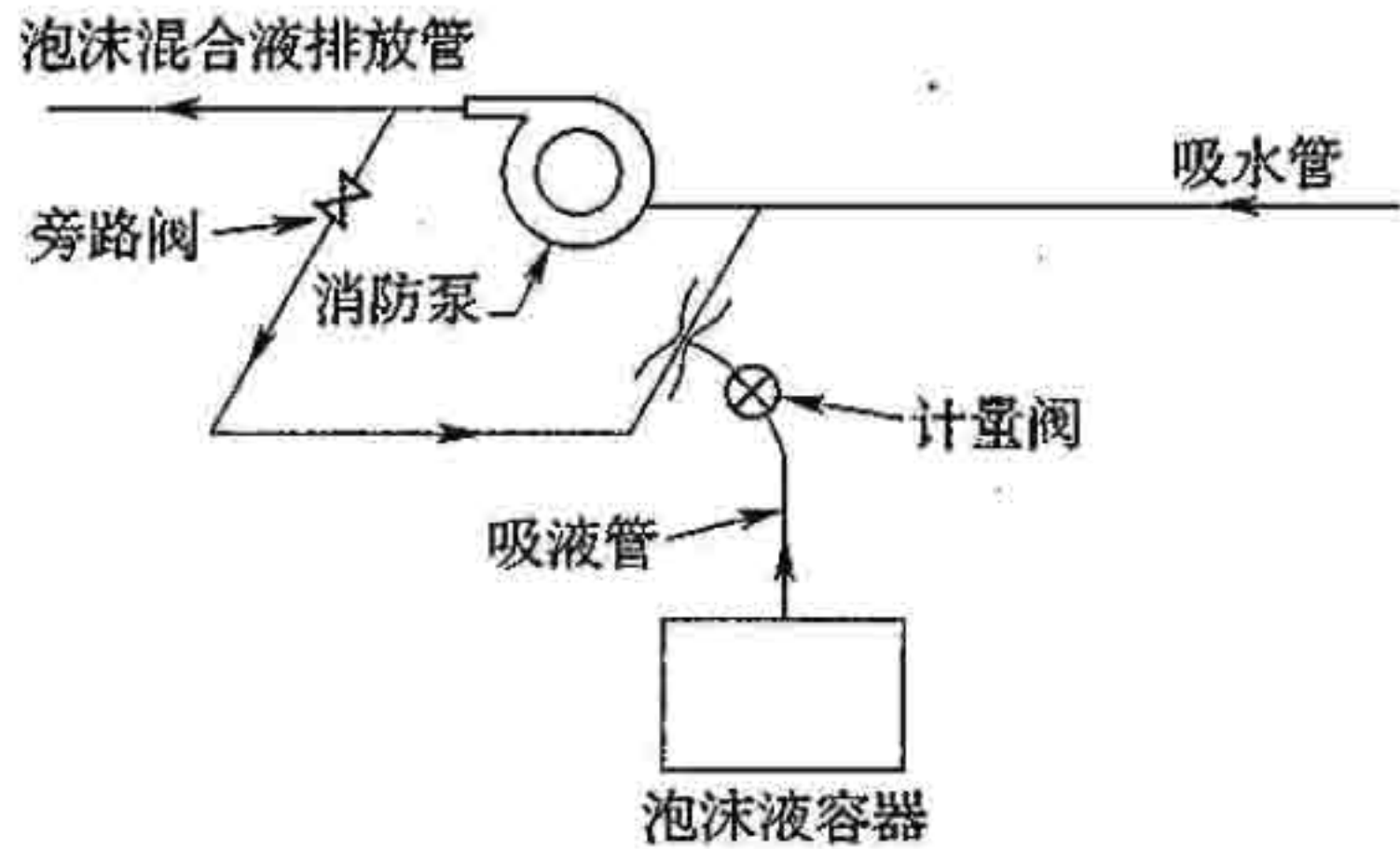
图 2 环泵式比例混合流程示意
